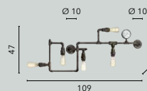
I-AMARCORD-PL5 8031440360487
