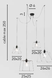
I-BROOKLYN-S4 8031414872282 4xE27
