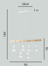
I-ARIZONA-S6 8031414872077 6xE27
