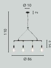
I-AMARCORD-S4 8031440360500
