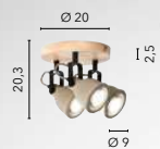
I-KISA-PL3 8031414897148 3xGU10
