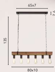
I-TEXAS-S6 8031414872008 6xE27
